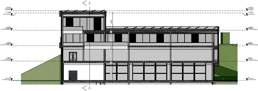
Doorsnede B-B
