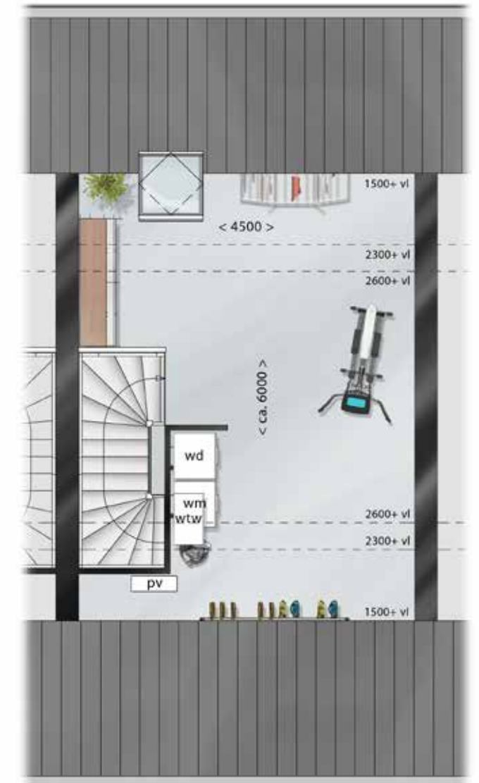
TWEDE VERDIEPING
