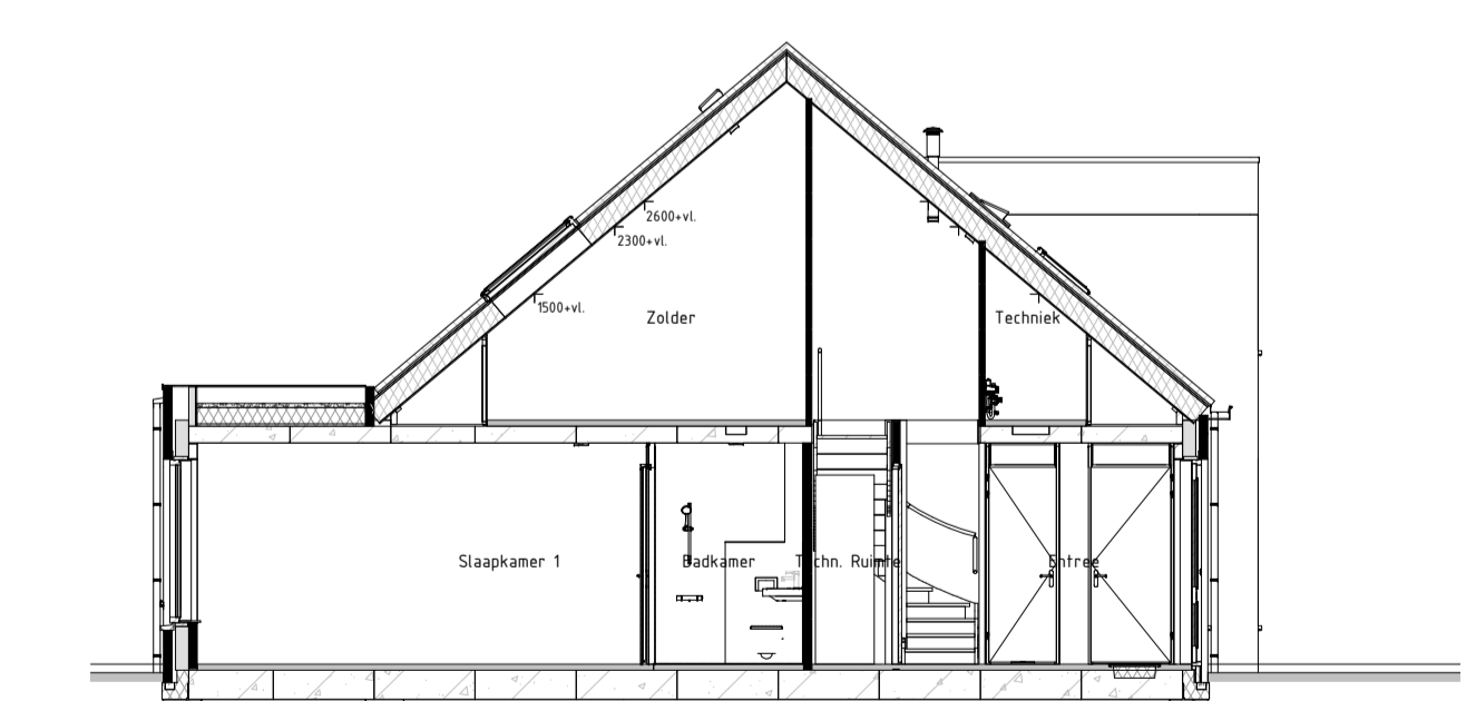
Doorsnede AA
