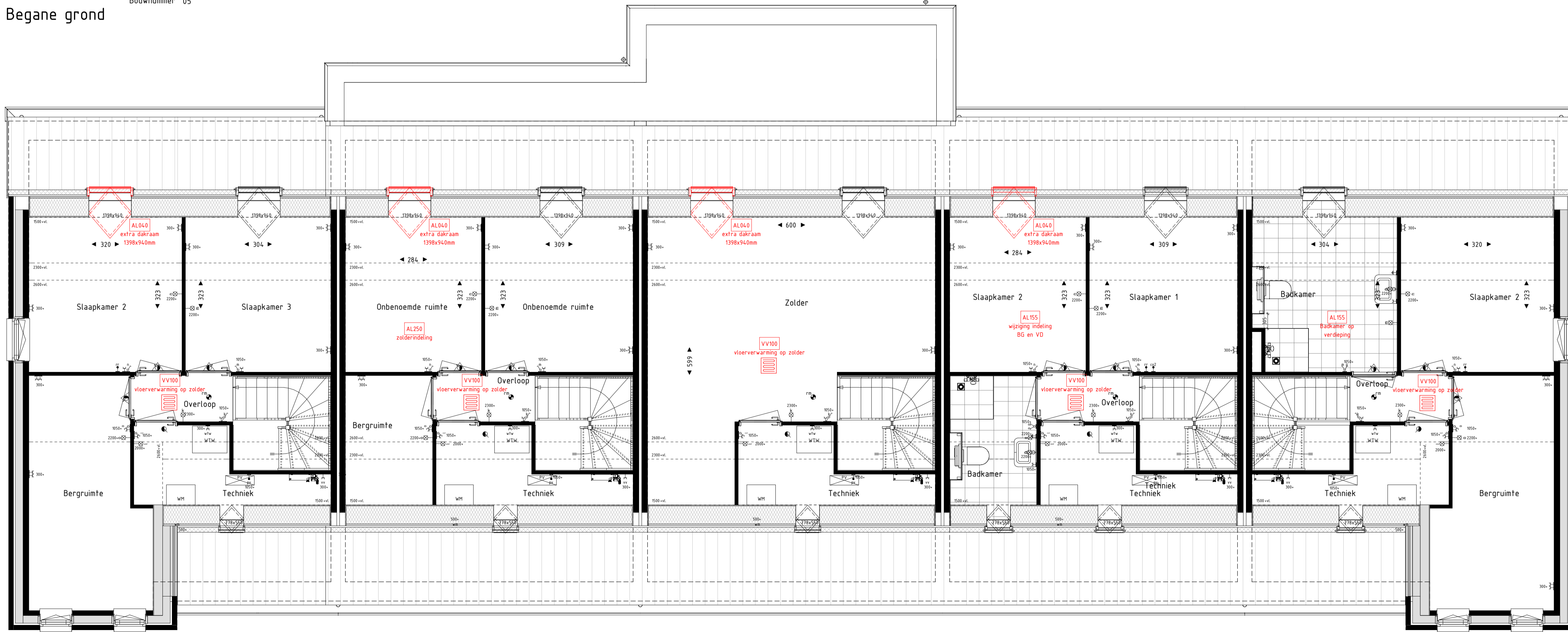
Eerste verdieping
