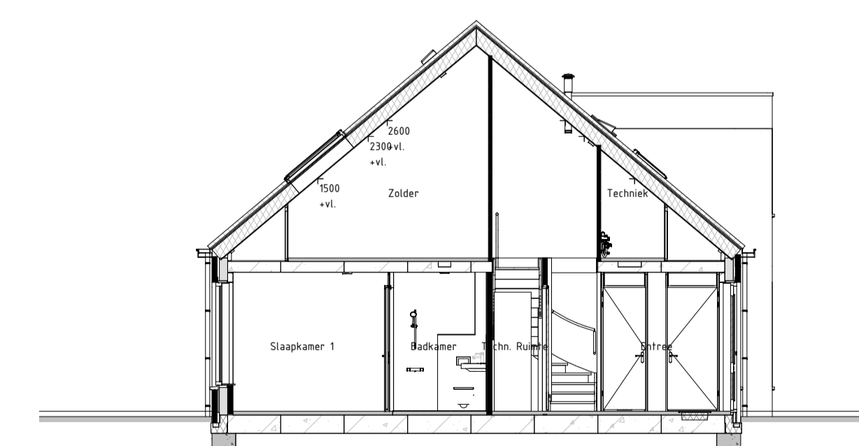
Doorsnede AA
