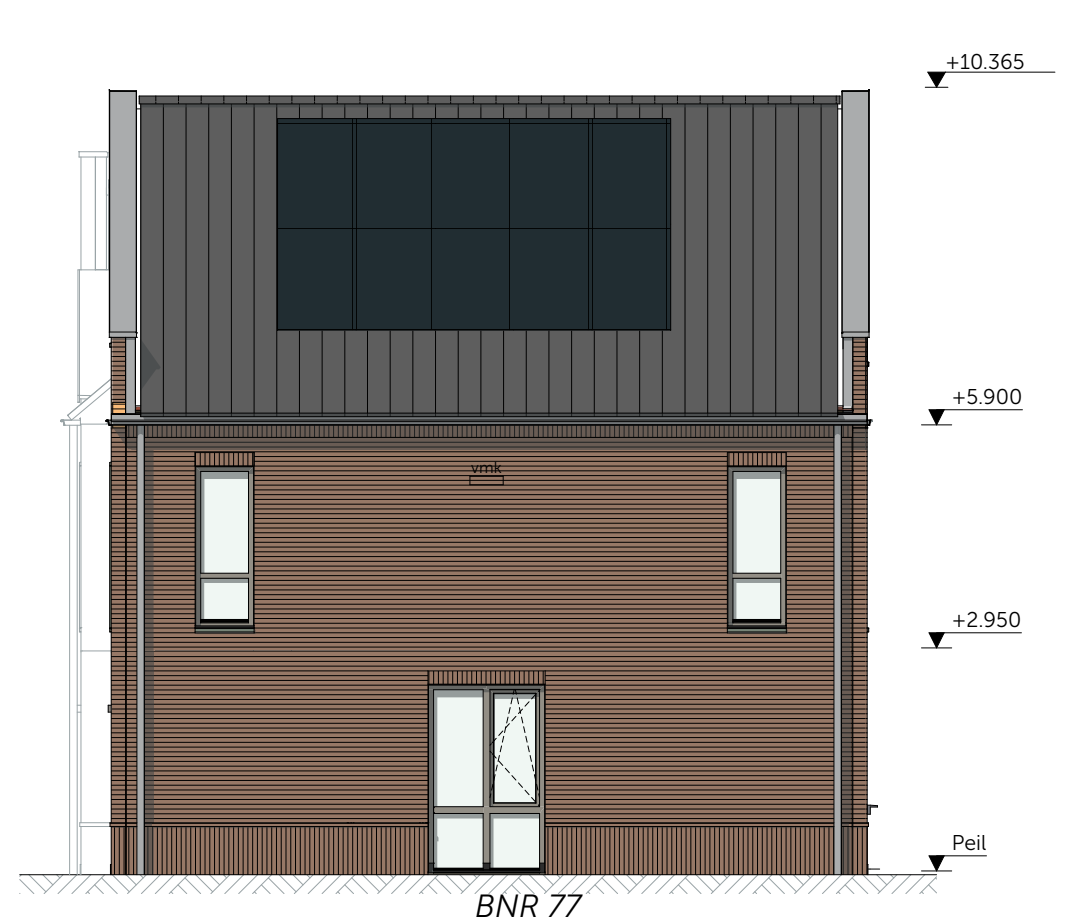
Rechtergevel - Blok 30 - Bruin schaal 1:100
