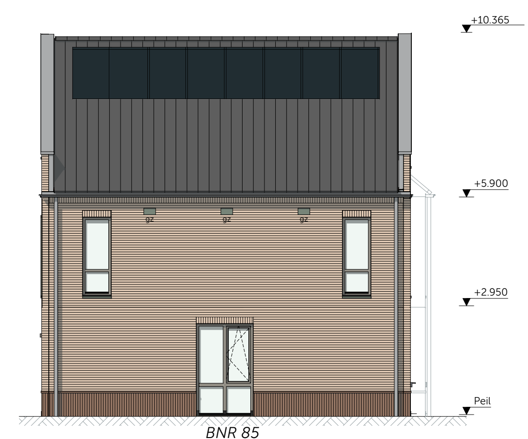
Rechtergevel - Blok 31 - Beige schaal 1:100
