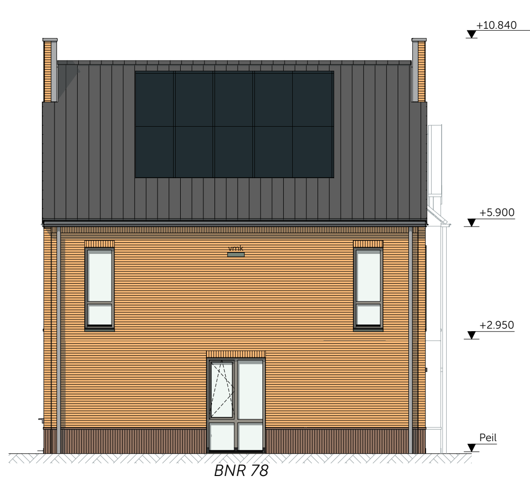
Linkergevel - Blok 31 - Oker schaal 1:100
