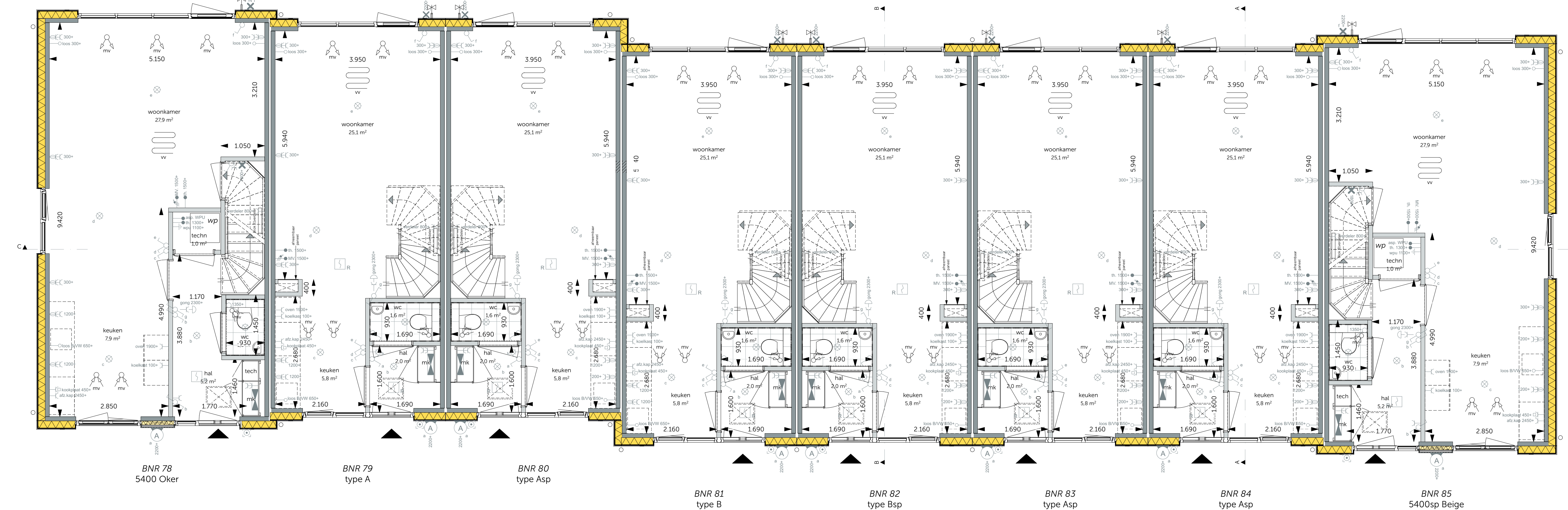
Begane grond schaal 1:50
