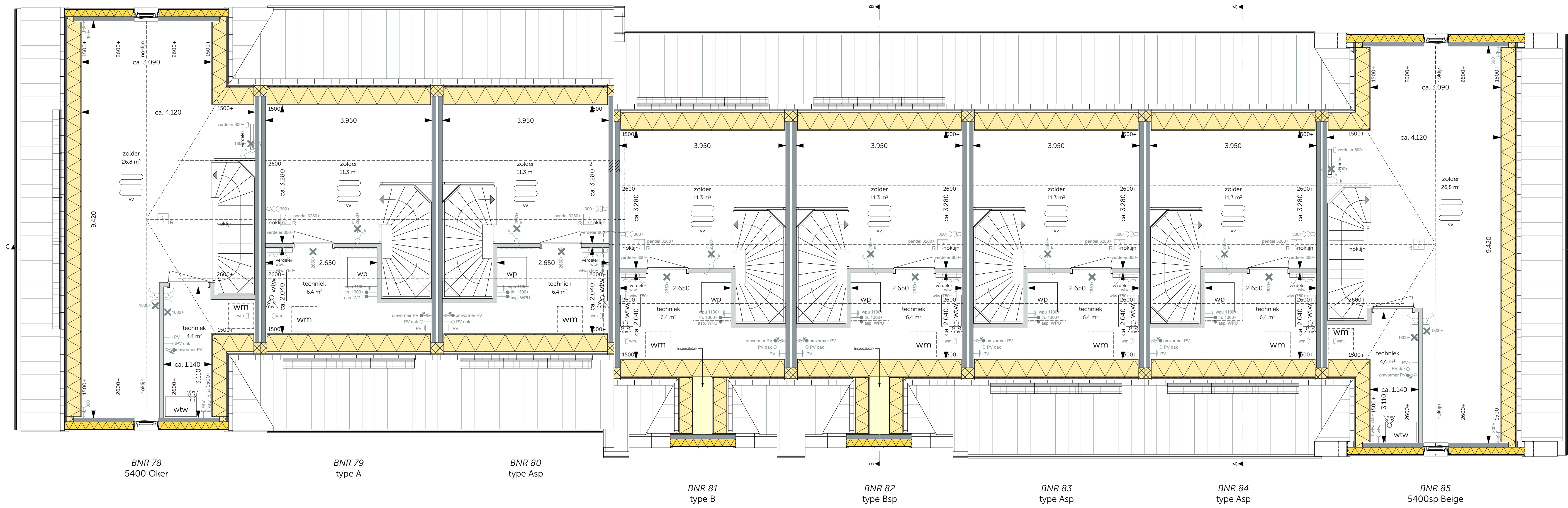
Tweede verdieping schaal 1:50
