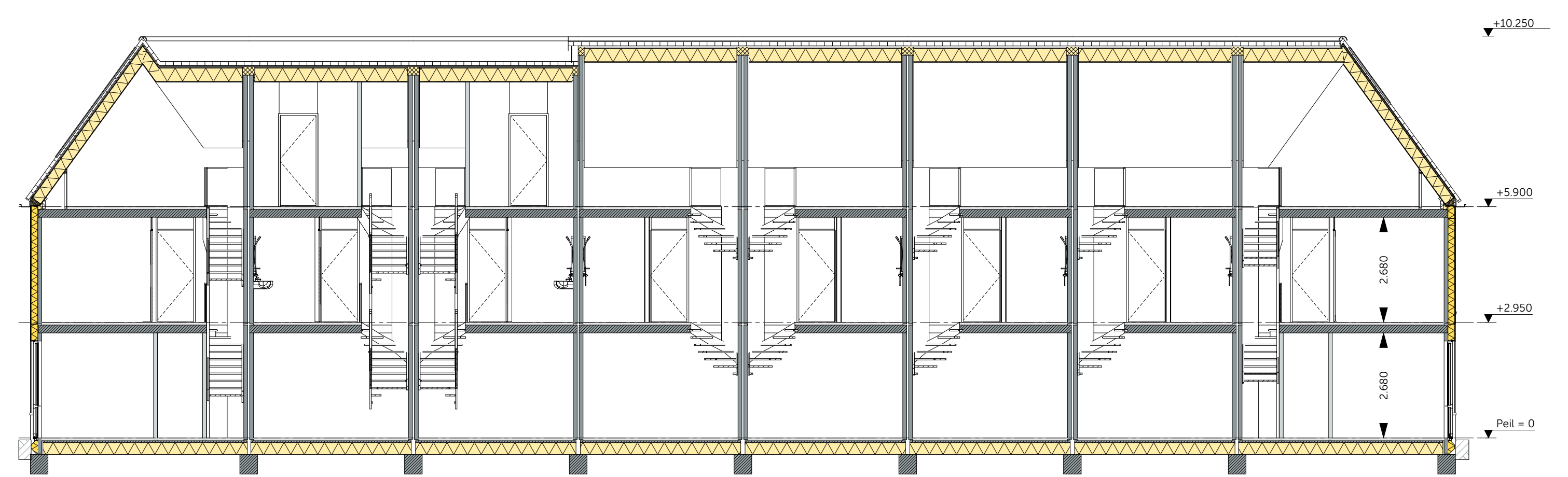
Doorsnede C-C schaal 1:100
