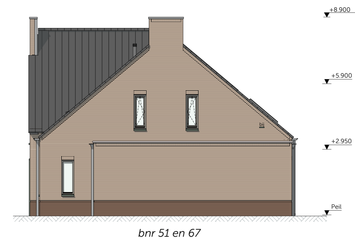
Rechtergevel schaal 1:100
