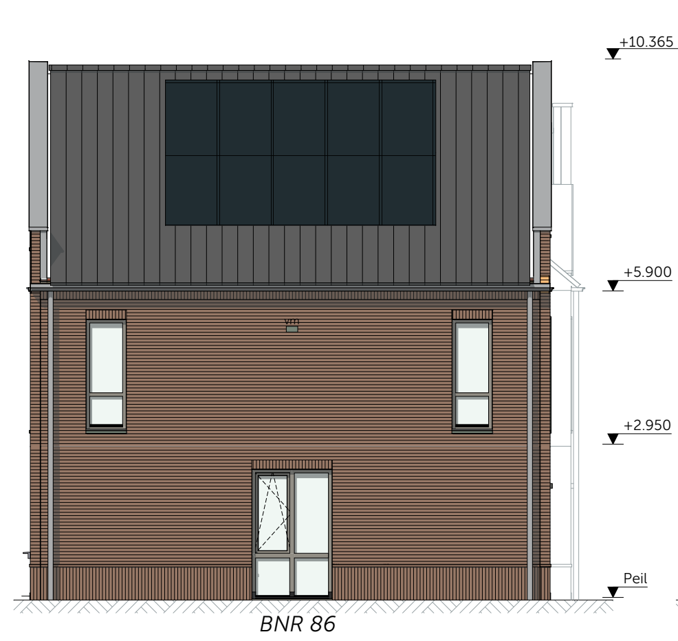
Linkergevel - Blok 32 - Bruin schaal 1:100
