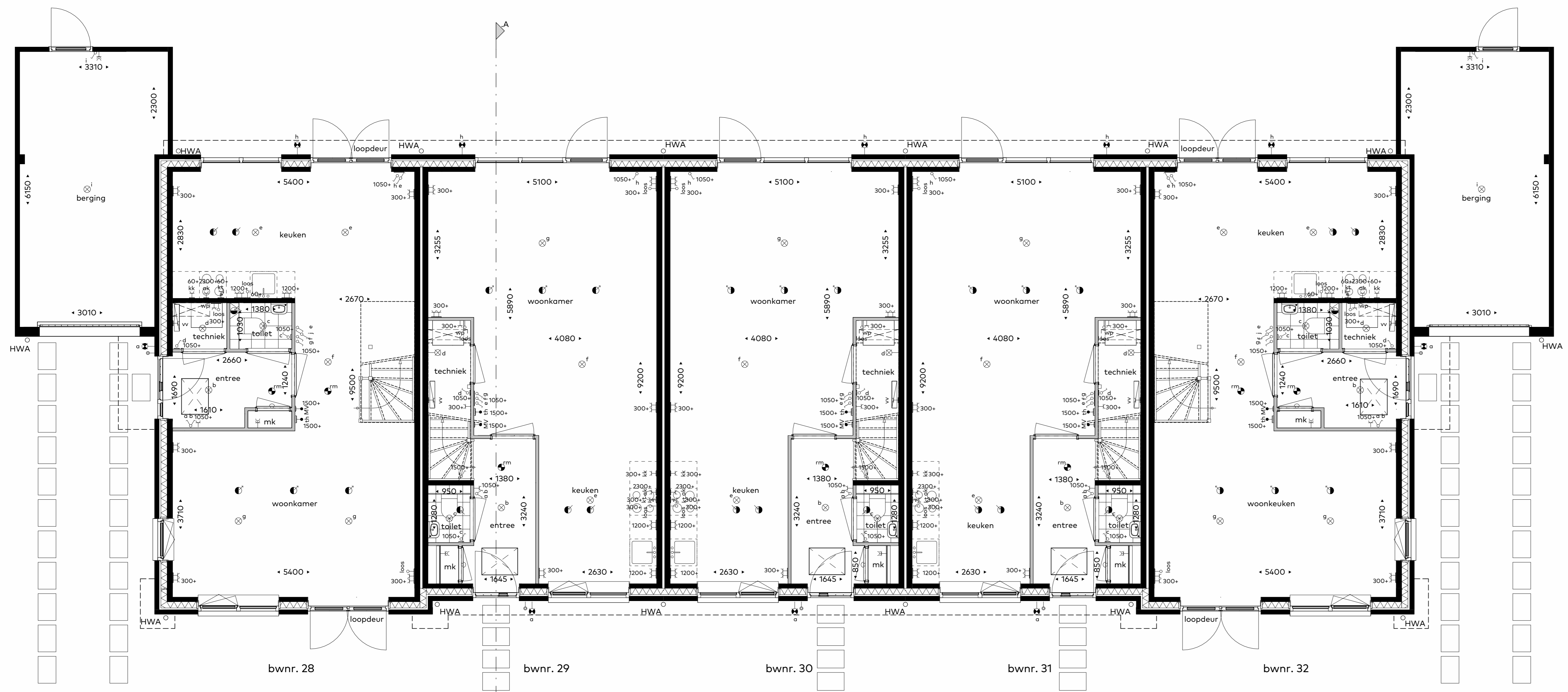
begane grond schaal 1:50
