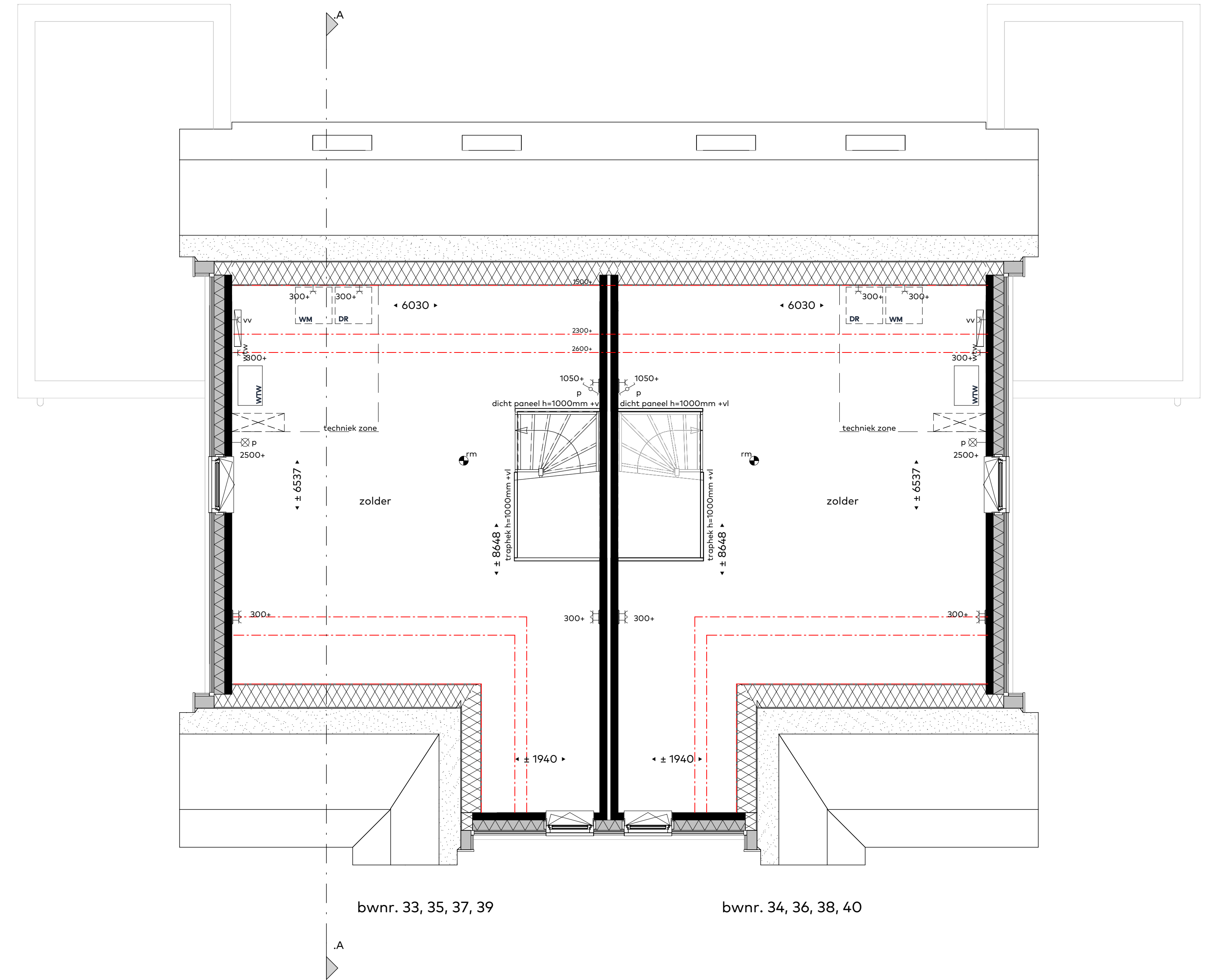
tweede verdieping schaal 1:50
