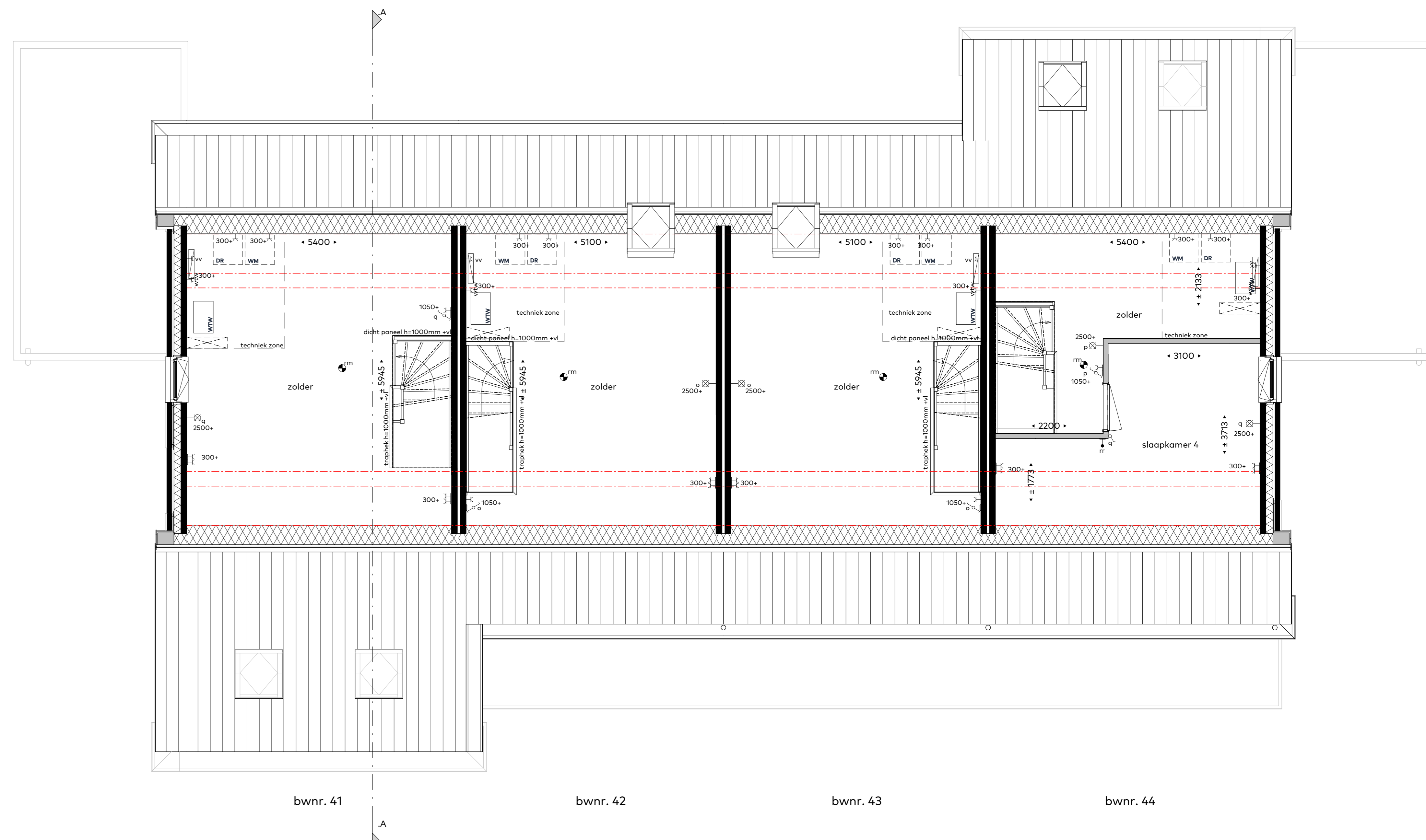
tweede verdieping schaal 1:50
