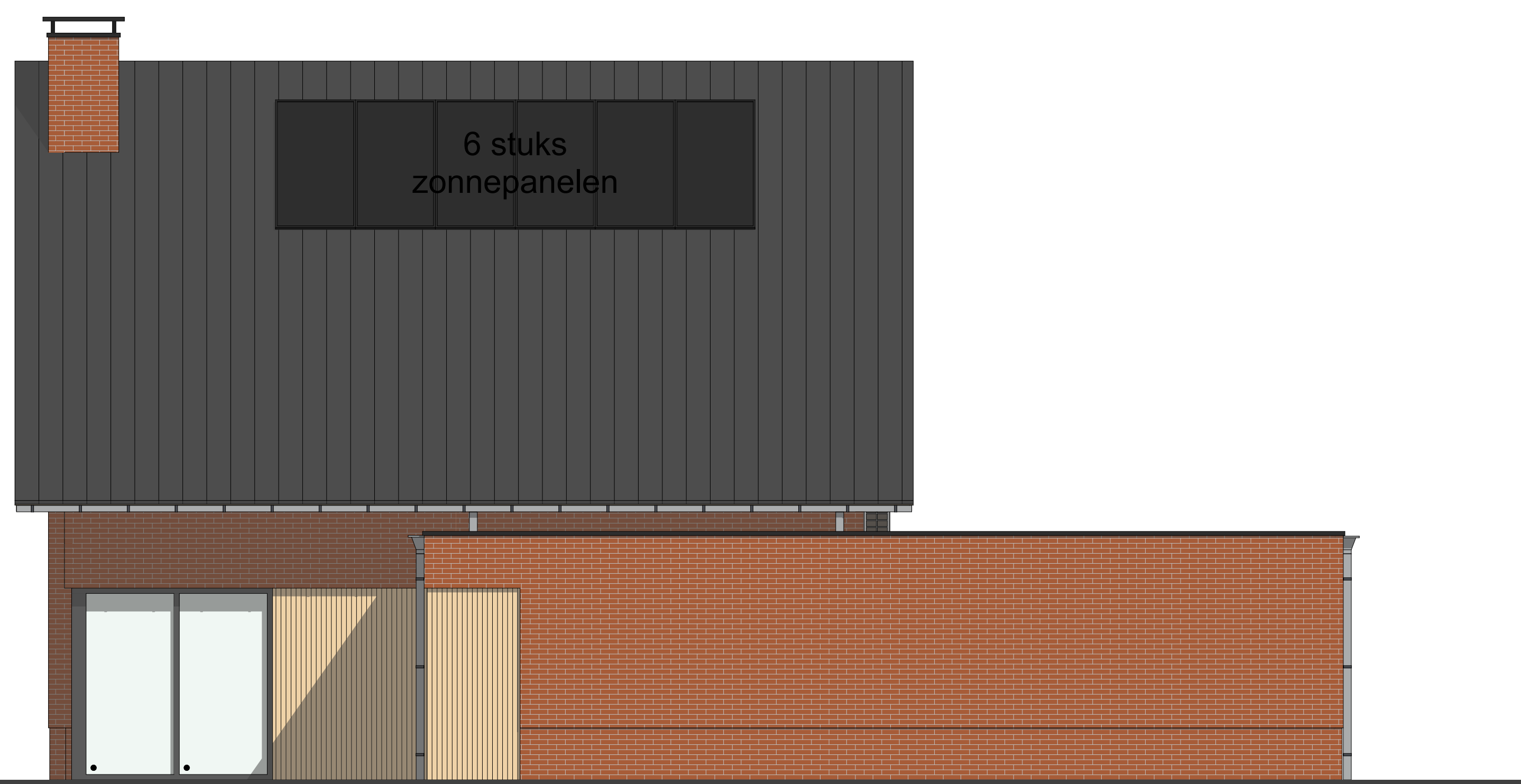
Rechtergevel
