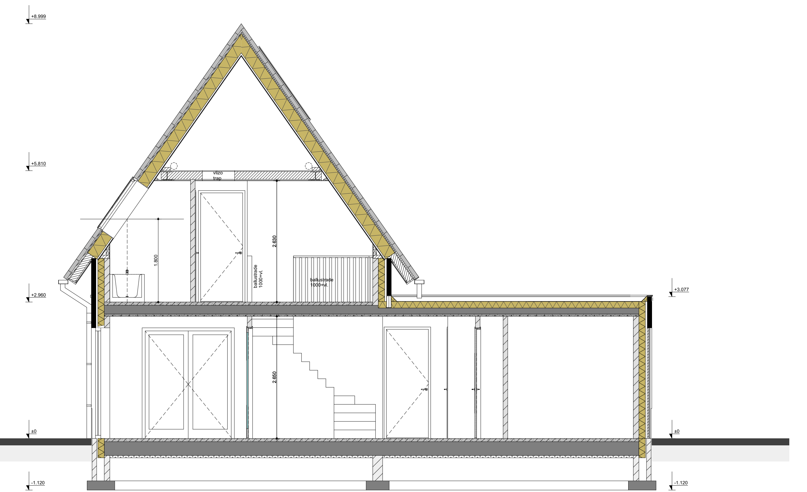
Doorsnede
