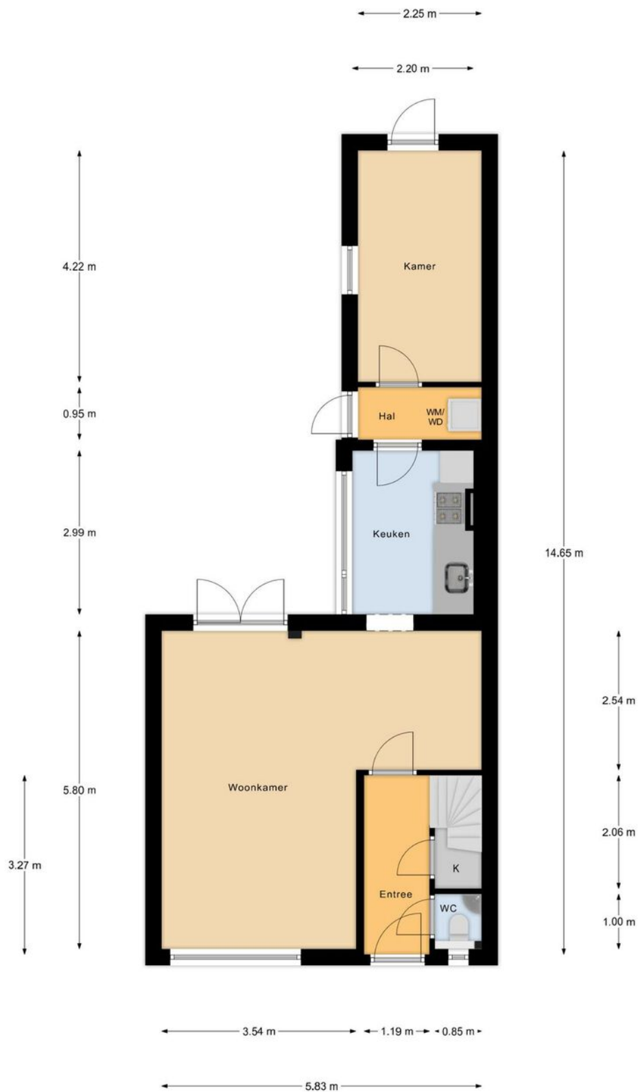
Begane Grond
