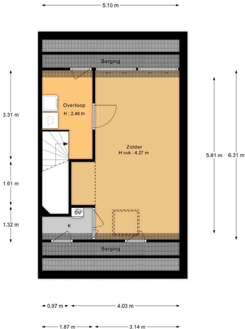
Tweede verdieping
