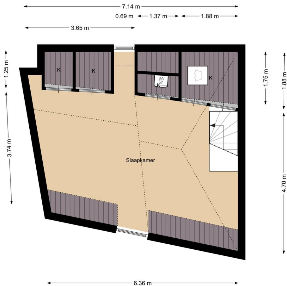
1e Verdieping
